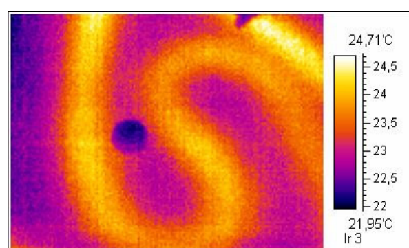
Kunststoff-FB-Heizungsrohr im Fußboden
